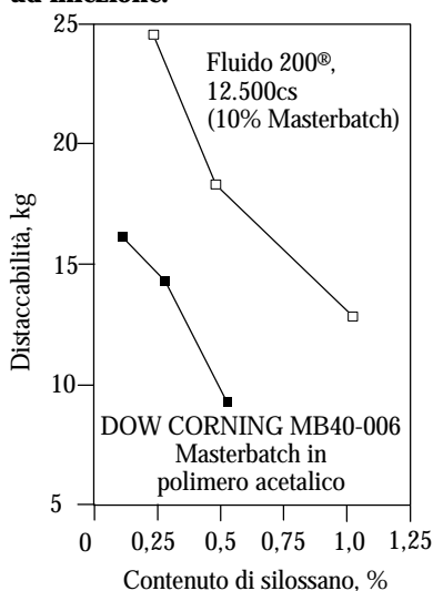
Figure 1: Effetto del silossano come agente di distacco nello stampaggio ad iniezione.
